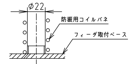
防振バネ部固定方法
