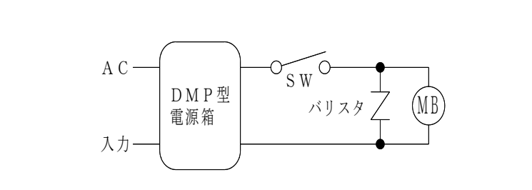
図3. 接続電気回路
