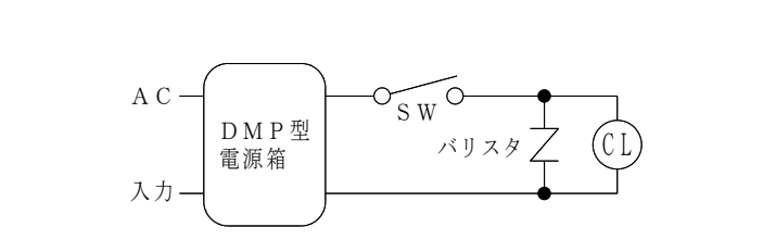
図 1．接続電気回路
