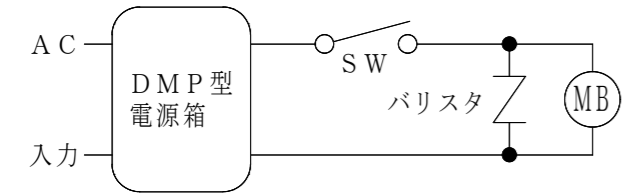
図 2. 接続電気回路
