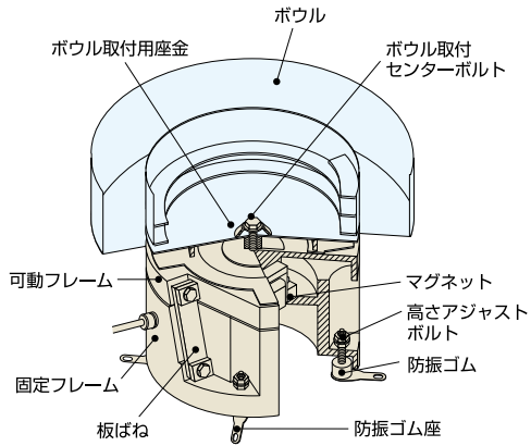
EA/ER構造図
