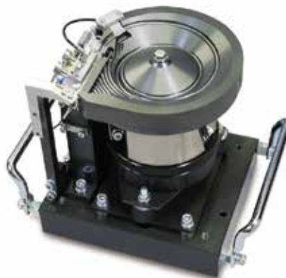
超薄物用パーツフィーダ
