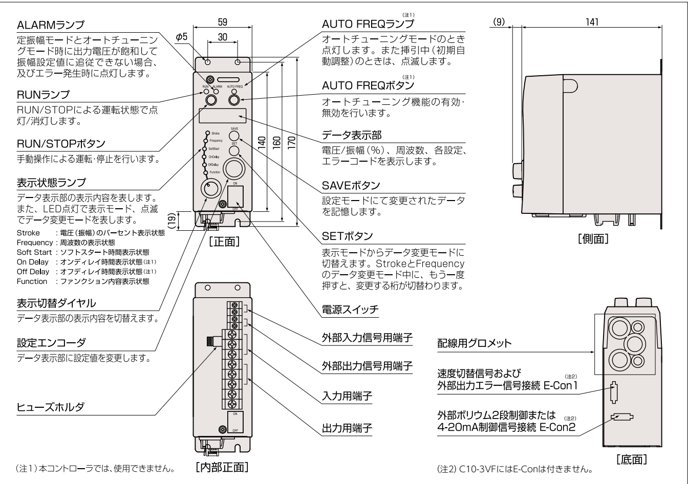
外形寸法図
