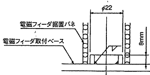
図2 据置バネ部位置固定方法
