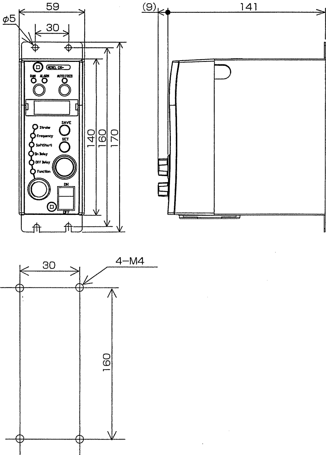
図4 コントローラ外形寸法
