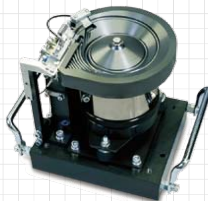
超薄材料零件供料机
