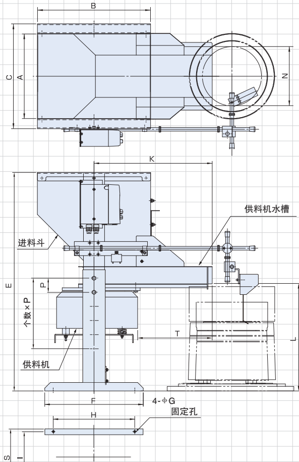
15/30/60/100 ℓ 进料斗 外形尺寸图
